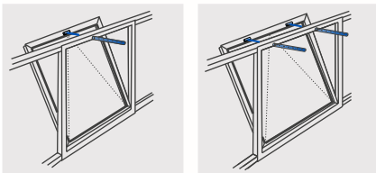
Верхнеподвесная створка
