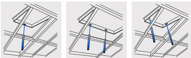
Зенитный фонарь
