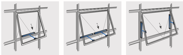
Верхнеподвесная опускаемая створка
